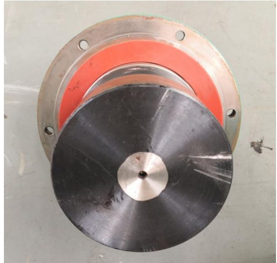
600 次手动松闸试验后的铁芯端面
